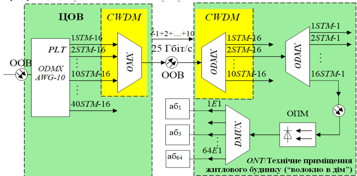
Рис. 1. Варіант застосування ВОСП CWDM в ОМД (напрявленя приймання).
