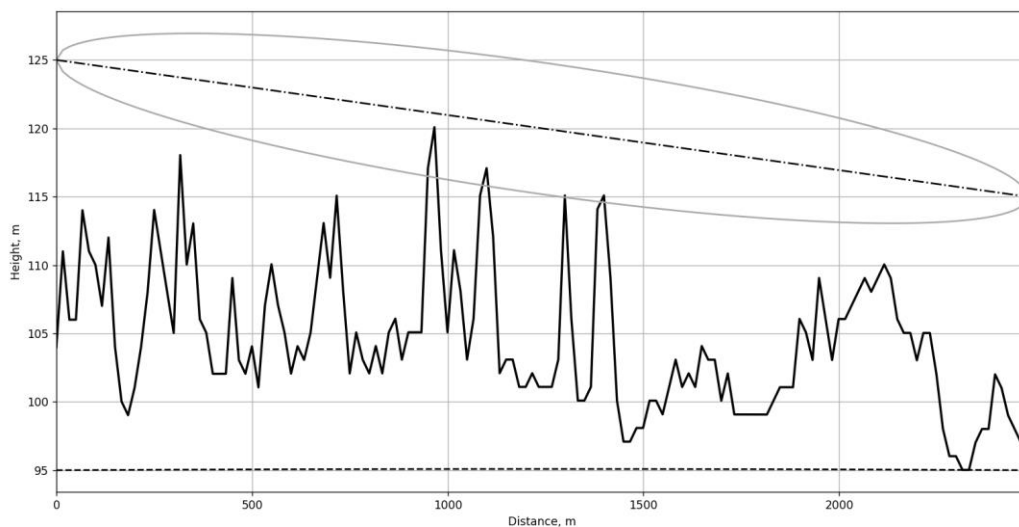
Рис.2. Графічна діаграма радіорелейного прольоту
