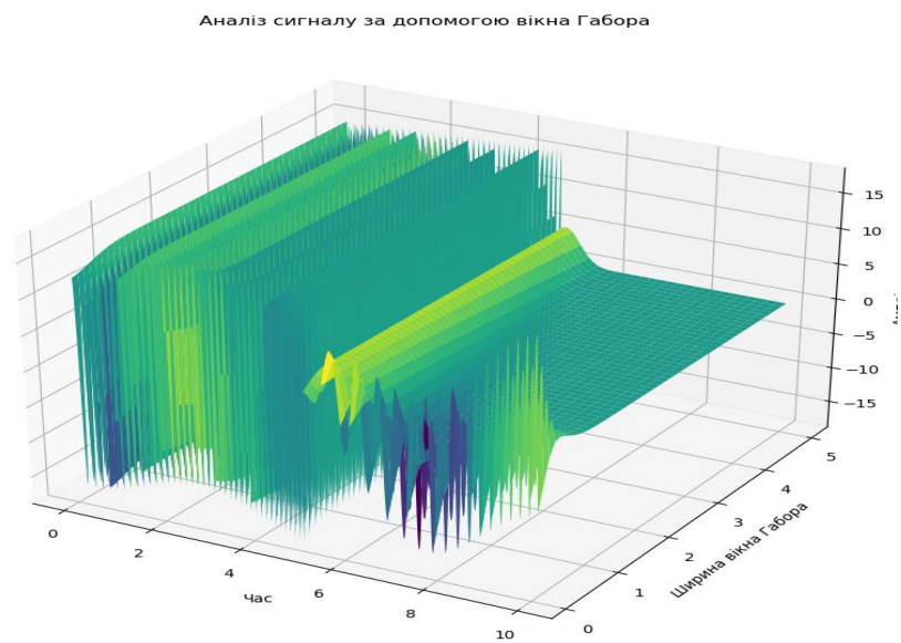
Рис.3. Вікно Габора.
