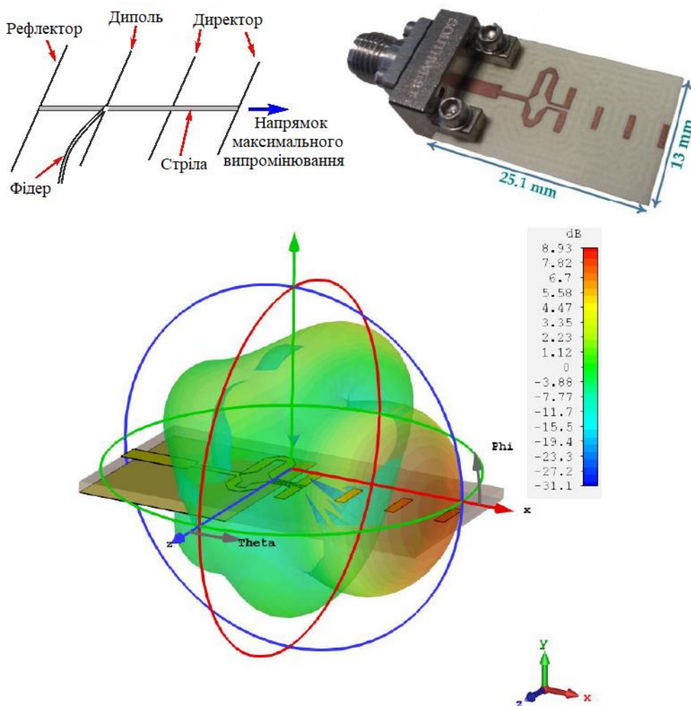
Рисунок 2. Антена Уда-Ягі та її діаграма Рисунок спрямованості.
