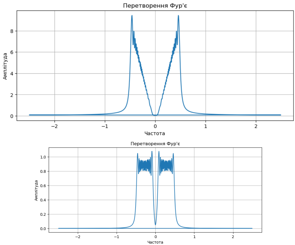
Рис.2. Перетворення Фур'є.
